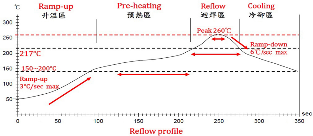
Lead-Free(LF)標準溫度分析範圍
