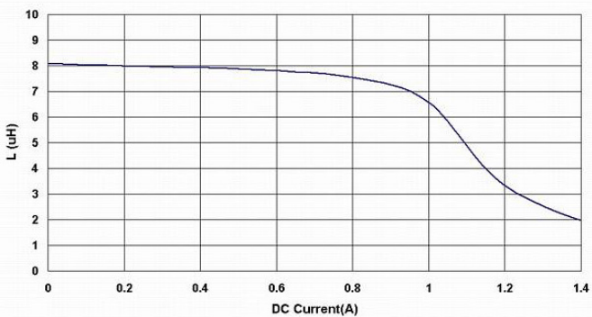
BPSC00050520101□S0
