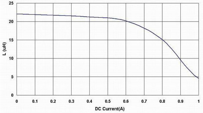
BPSC00050520270□S0
