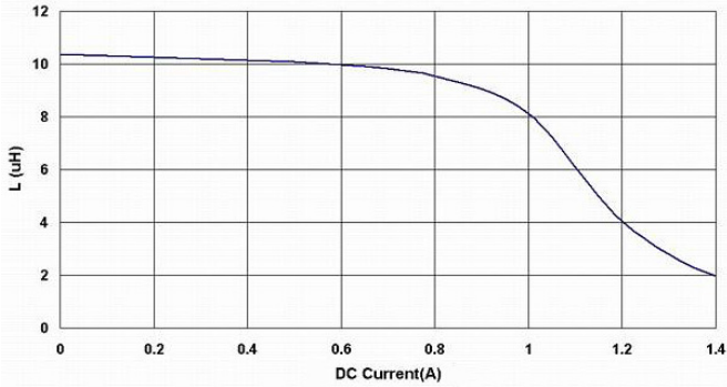
BPSC00050520120□S0
