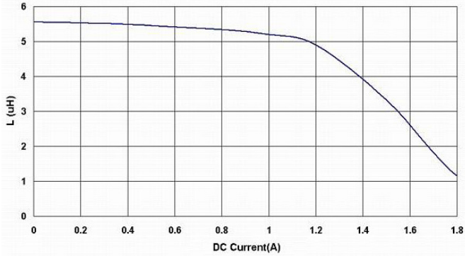
BPSC000505206R8□S0
