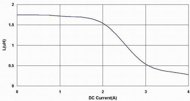
BPSC000505202R2□S0
