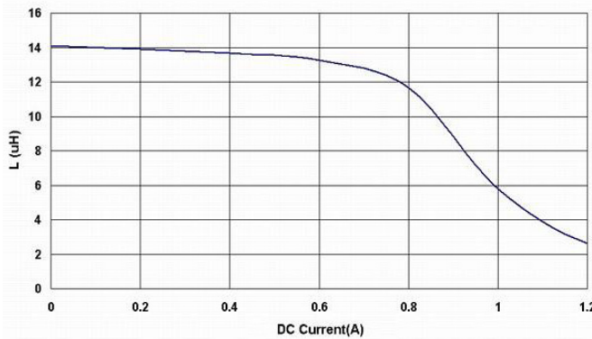
BPSC00050520180□S0
