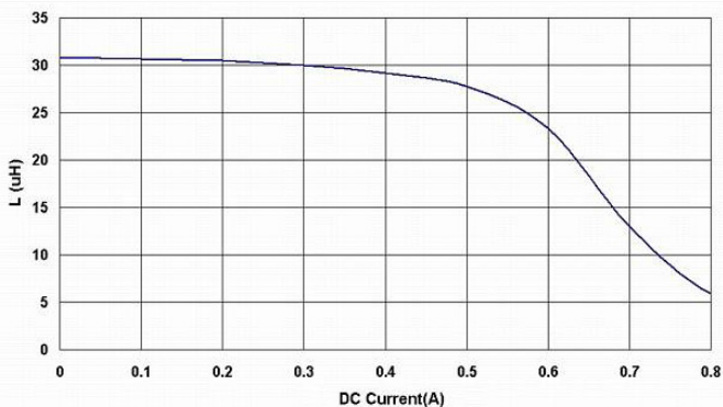
BPSC00050520390□S0
