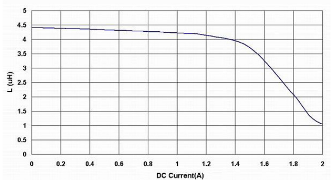
BPSC000505204R7□S0
