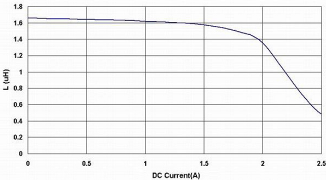
BPSC000505201R8□S0
