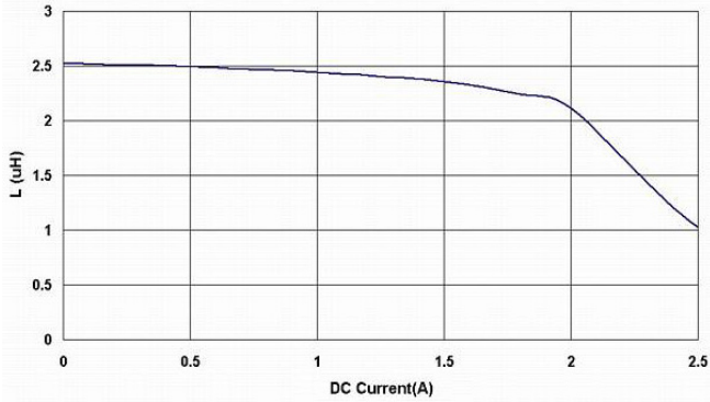
BPSC000505203R3□S0
