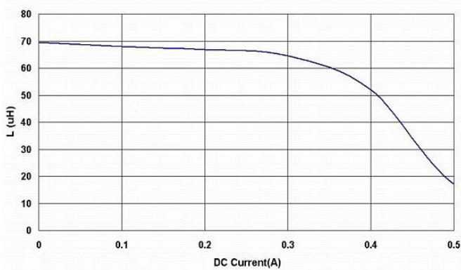
BPSC00050520680□S0
