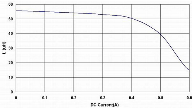
BPSC00050520680□S0
