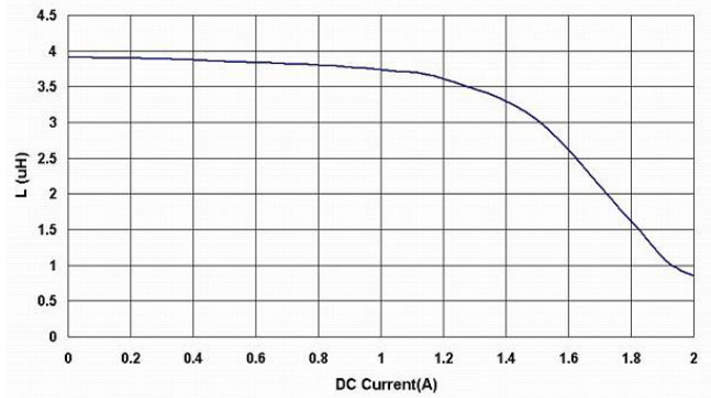
BPSC000505204R7□S0
