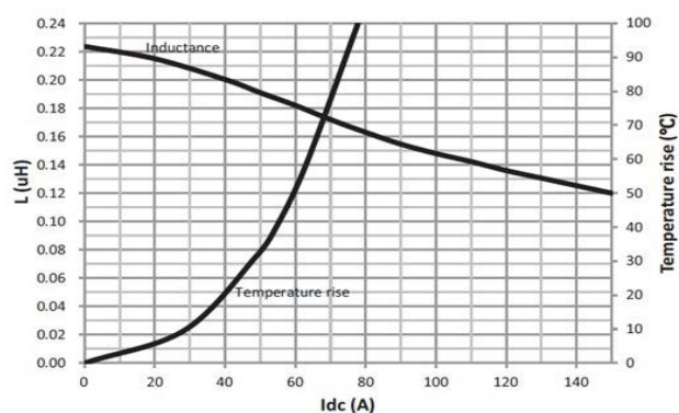
HCM1A1305V3-R22-R
