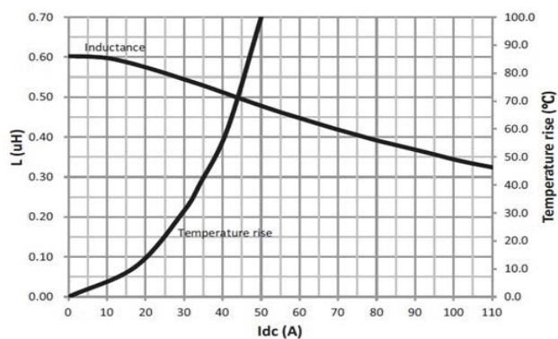
HCM1A1305V3-R56-R
