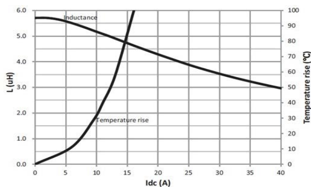
HCM1A1305V3-5R6-R
