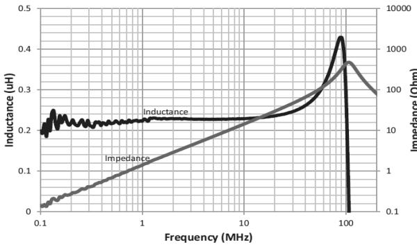
HCM1A1305V3-R22-R
