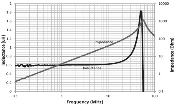
HCM1A1305V3-R56-R
