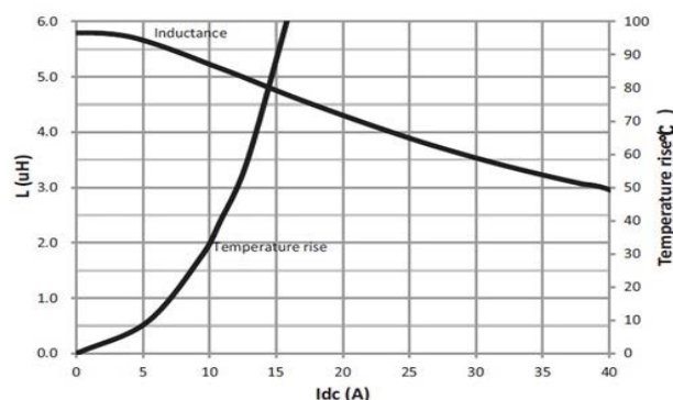
HCM1A1305V3-6R0-R
