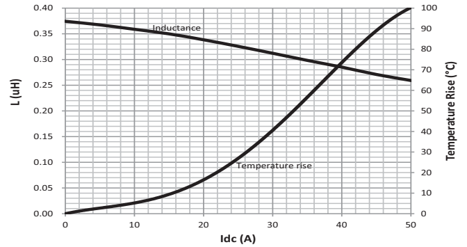
HCM1A1104V3-R36-R
