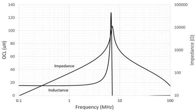
HCM1A1104V3-150-R
