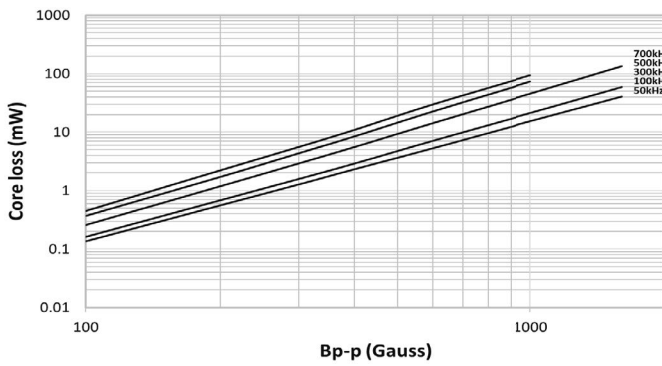
HCM1A1104V3-150-R
