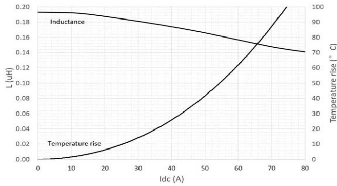
HCM1A1104V3-R20-R
