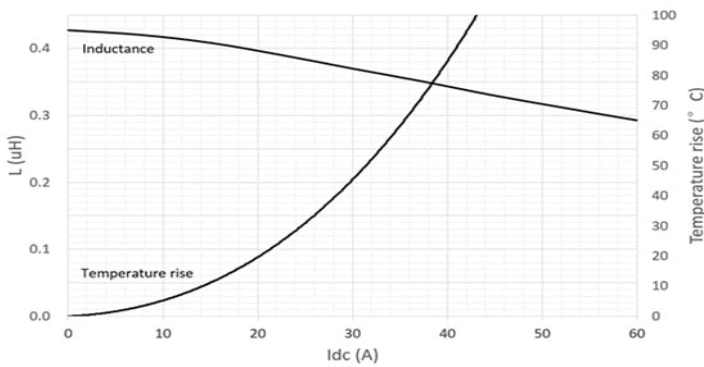
HCM1A1104V3-R45-R
