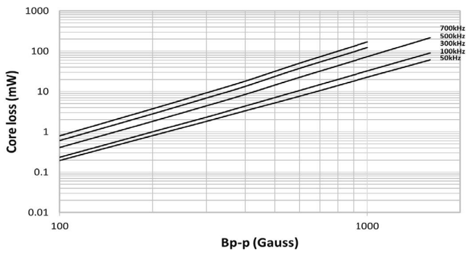
HCM1A1104V3-R20-R
