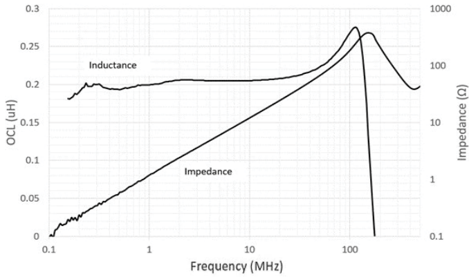
HCM1A1104V3-R20-R
