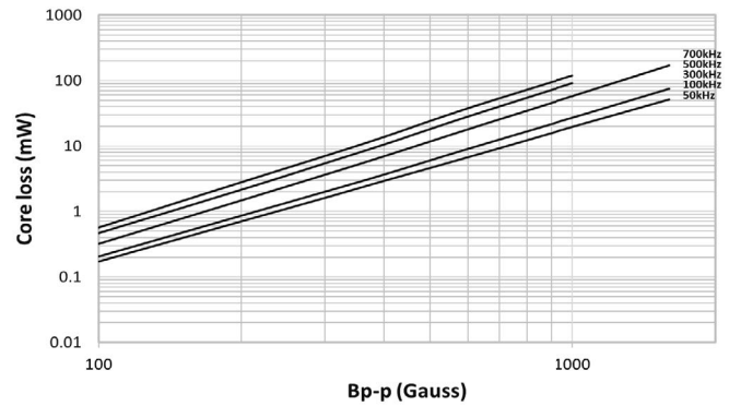
HCM1A1104V3-5R6-R
